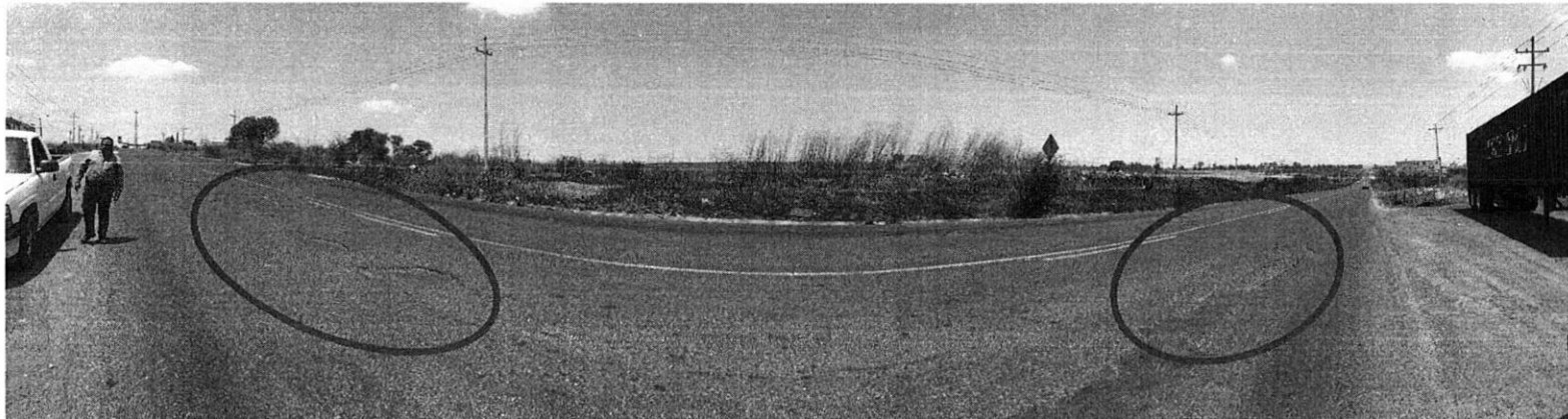
Carpeta de concreto asfáltico en caliente, ubicado entre los municipios de San Juan de los Lagos y Encarnación de Díaz, en la localidad de El Desperdicio, que presenta daños, baches y desgaste propio del uso y del intemperismo.
