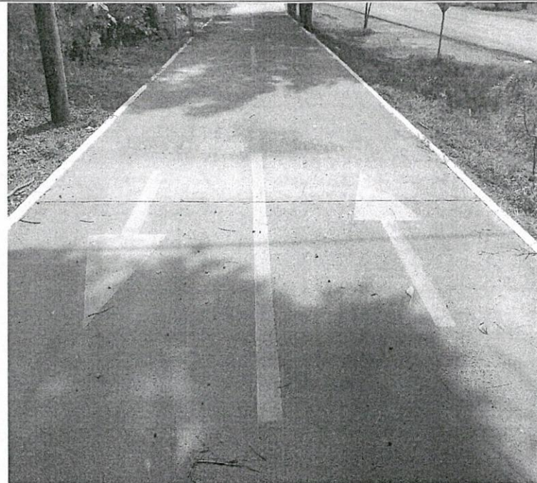
"Construcción de Ciclovía a base de Banqueta de Concreto F'C= 150 Kg/Cm2 de 8 cm. de espesor, Machuelos, Señalética, Luminarias LEDS y Construcción de "Cajas" Guardabicicletas"
